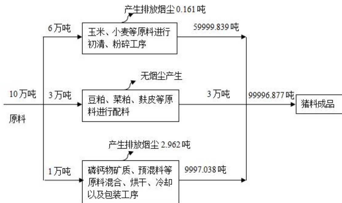
（3） 扩建前猪料生产线物料平衡图
