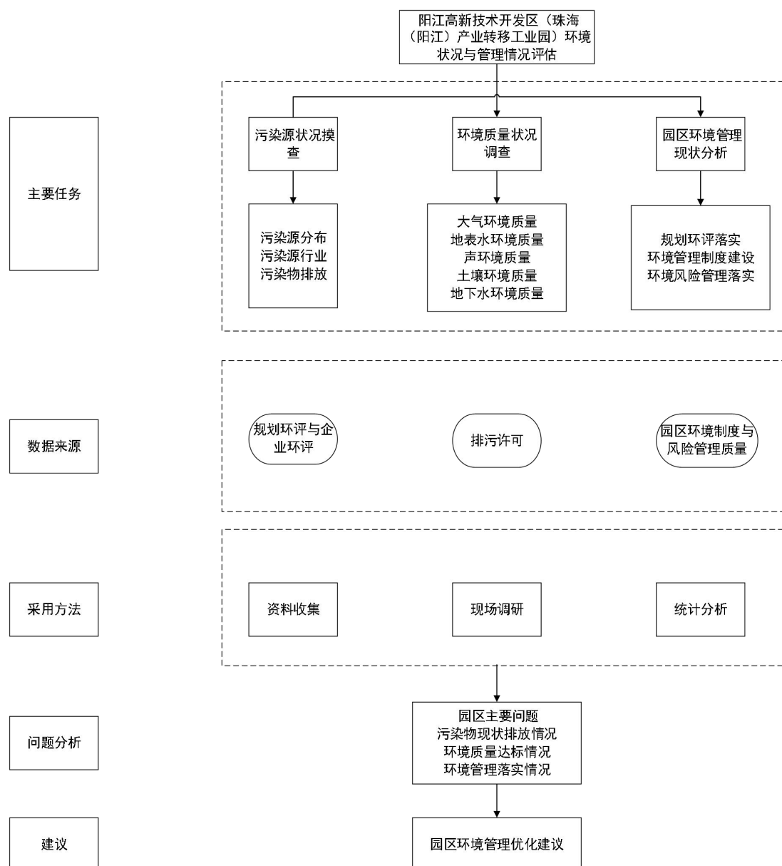
图 1.7-1 技术路线图
